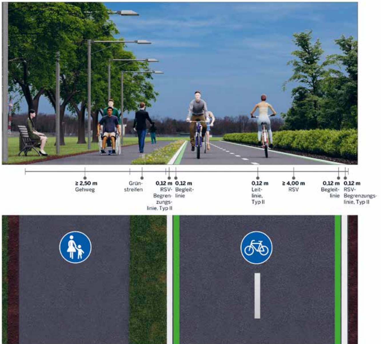
Abbildung 2: Eigenständig geführte RSV im Zweirichtungsverkehr, Trennung durch Grünstreifen (Skizze)
